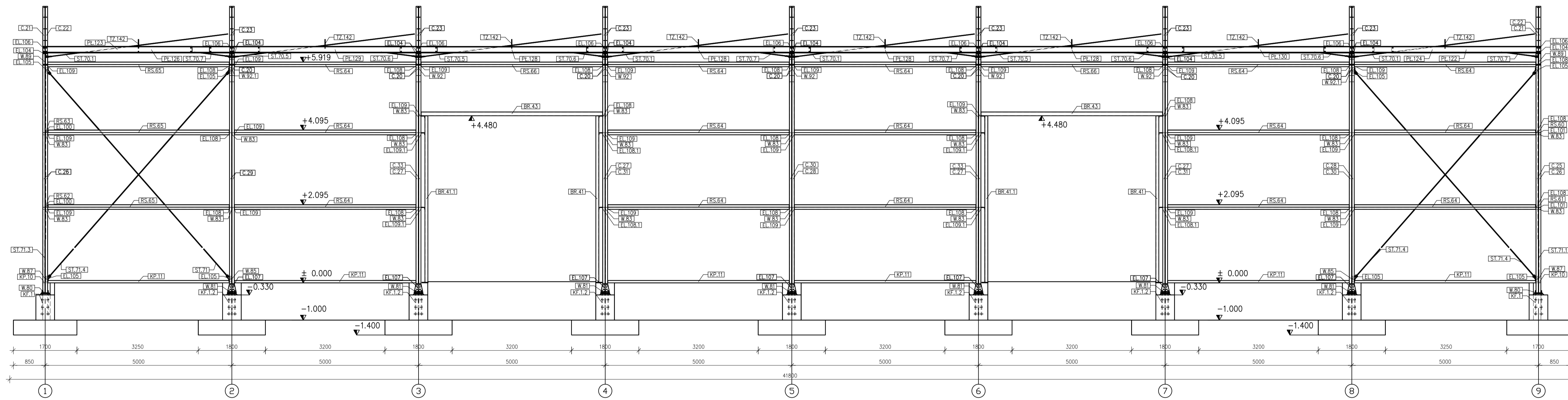
Przekrój w osi "C"(Sc1:50)
